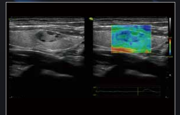
Thyroid EI
